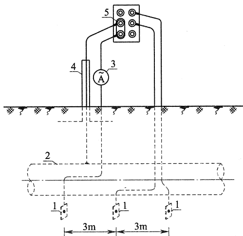
图 A.3.2 交流电流密度测量接线图
